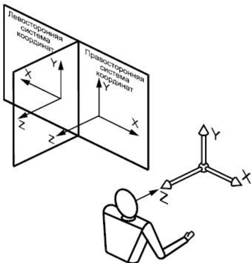
Рисунок 1 - Система координат
